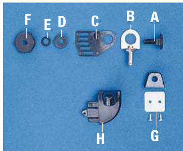
Accesorio de liberación instantánea
